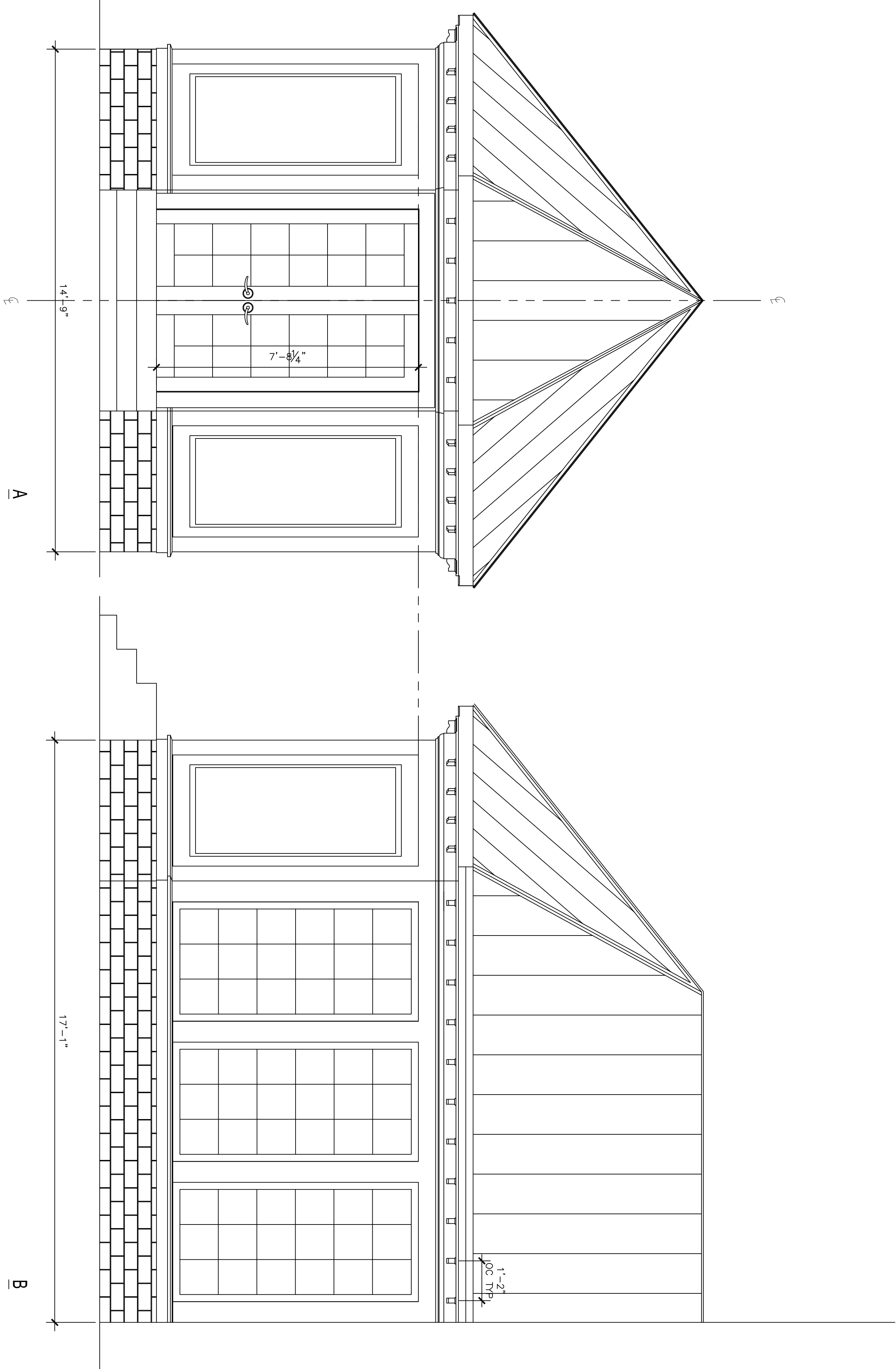
2 ELEVATION SCALE: 1/2" = 1'-0"
